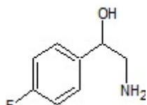
2-Amino-1-(4-fluorophenyl) ethanol
